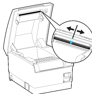
Printera tīrīšana
