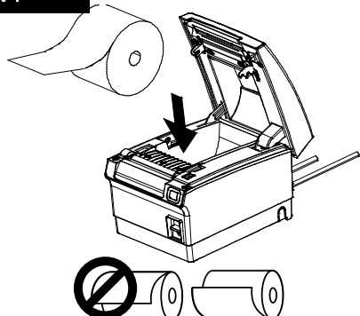
Εγκατάσταση χαρτιού 2
