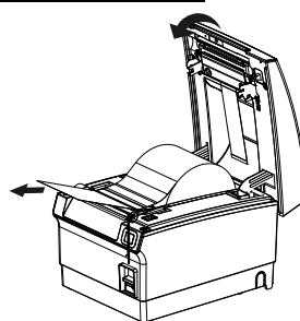
Namestitev papirja 5
