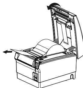
Εγκατάσταση χαρτιού 5
