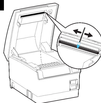
Čiščenje tiskalnika
