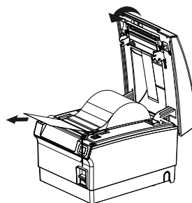
Papīra ievietošana 5
