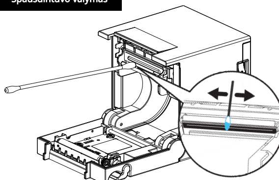
Spausdintuvo valymas
