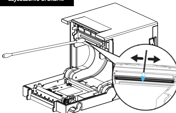
Czyszczenie drukarki
