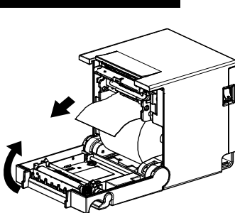
Installazione della carta 3
