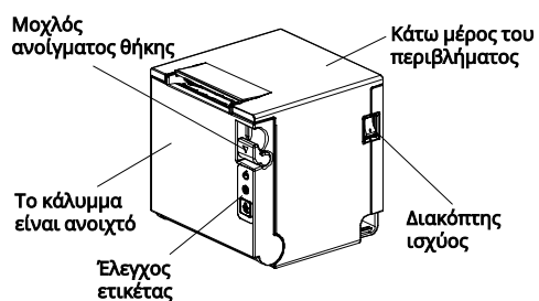
Όνομα εξαρτημάτων
