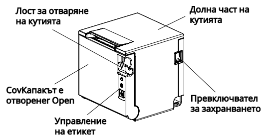
Имена на частите
