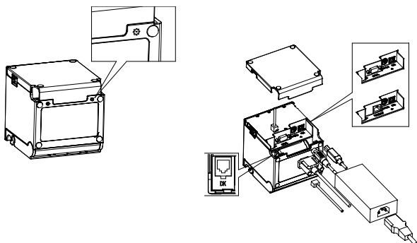
Paperin asennus 1
