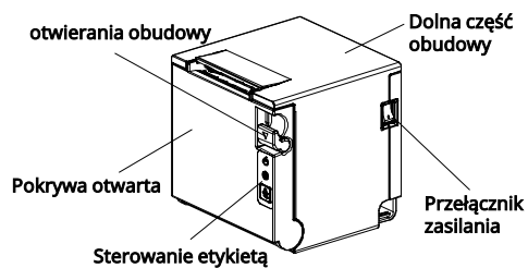
Nazwa części
