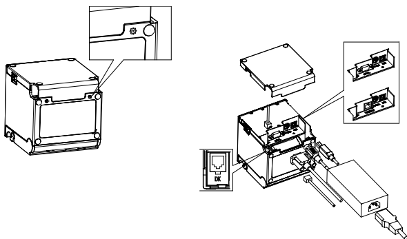
Εγκατάσταση χαρτιού 1
