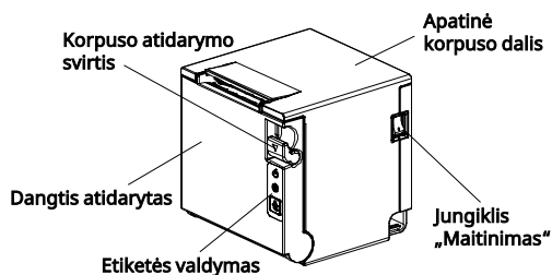
Dalių pavadinimas
