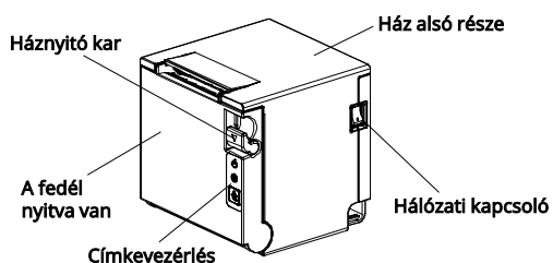
Alkatrészek neve
