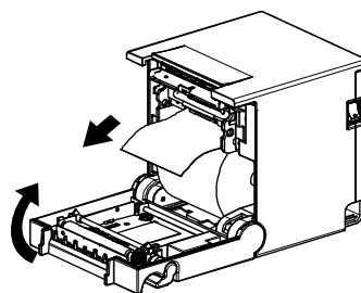
Popieriaus montavimas 5
