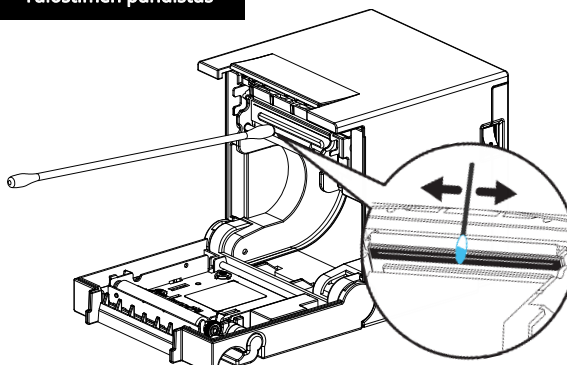
Tulostimen puhdistus
