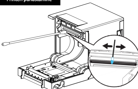
Printeri puhastamine
