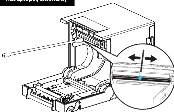
Καθαρισμός εκτυπωτή
