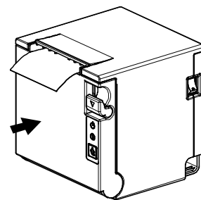
Namestitev papirja 4
