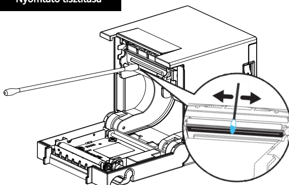
Nyomtató tisztítása
