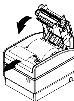
Инсталиране на преграда
