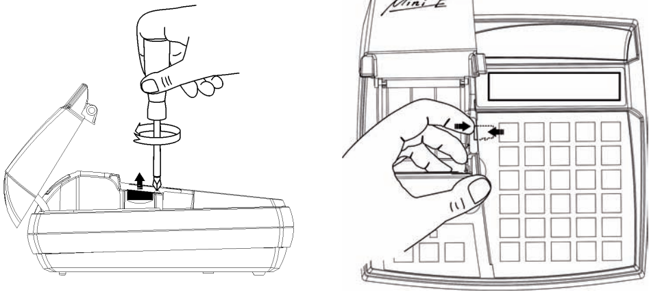
Rys. 3-1 Umieszczenie karty w kasie i sposób jej wyjmowania
