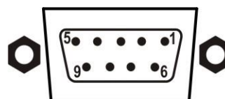
Rys. 8-8 Terminal Płatniczy (DSUB9 wtyk)
