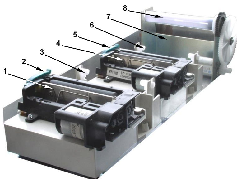
Rys. 2-6 Budowa zespołu drukującego
