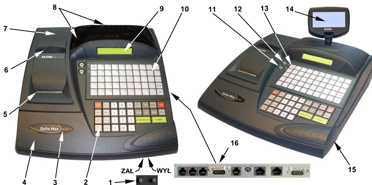
Rys. 1-1 Widok kasy
